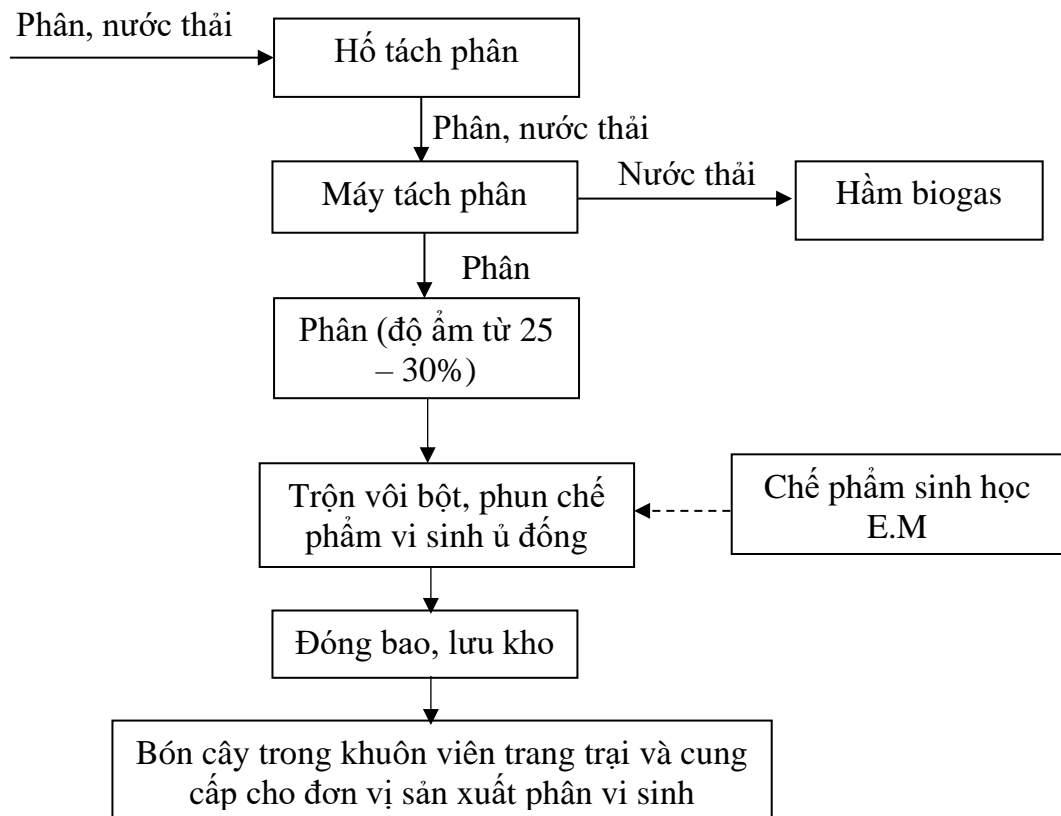
Hình 3.22: Sơ đồ thu gom phân của trang trại
