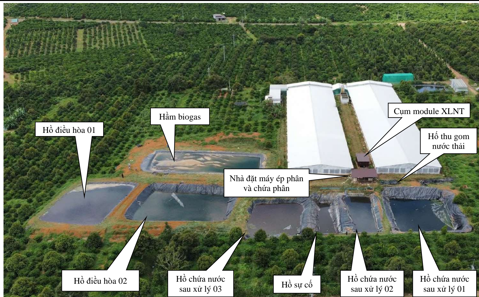
Hình 3.9: Hình ảnh hệ thống xử lý nước thải tập trung của trang trại
