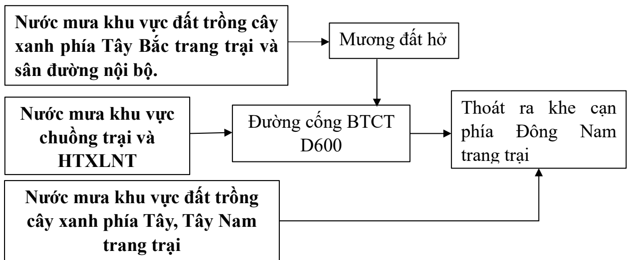
Hình 3.2: Sơ đồ hệ thống thu gom và thoát nước mưa của trang trại
