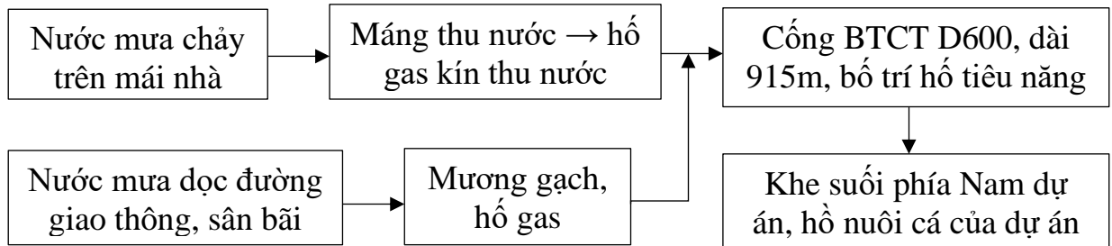
Hình 3.1: Sơ đồ hệ thống thu gom và thoát nước mưa của trang trại theo ĐTM
