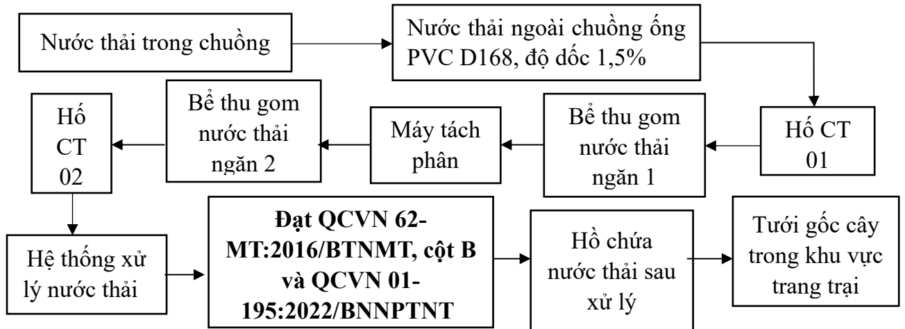
Hình 3.6: Sơ đồ mạng lưới thu gom và tái sử dụng nước thải của trang trại
