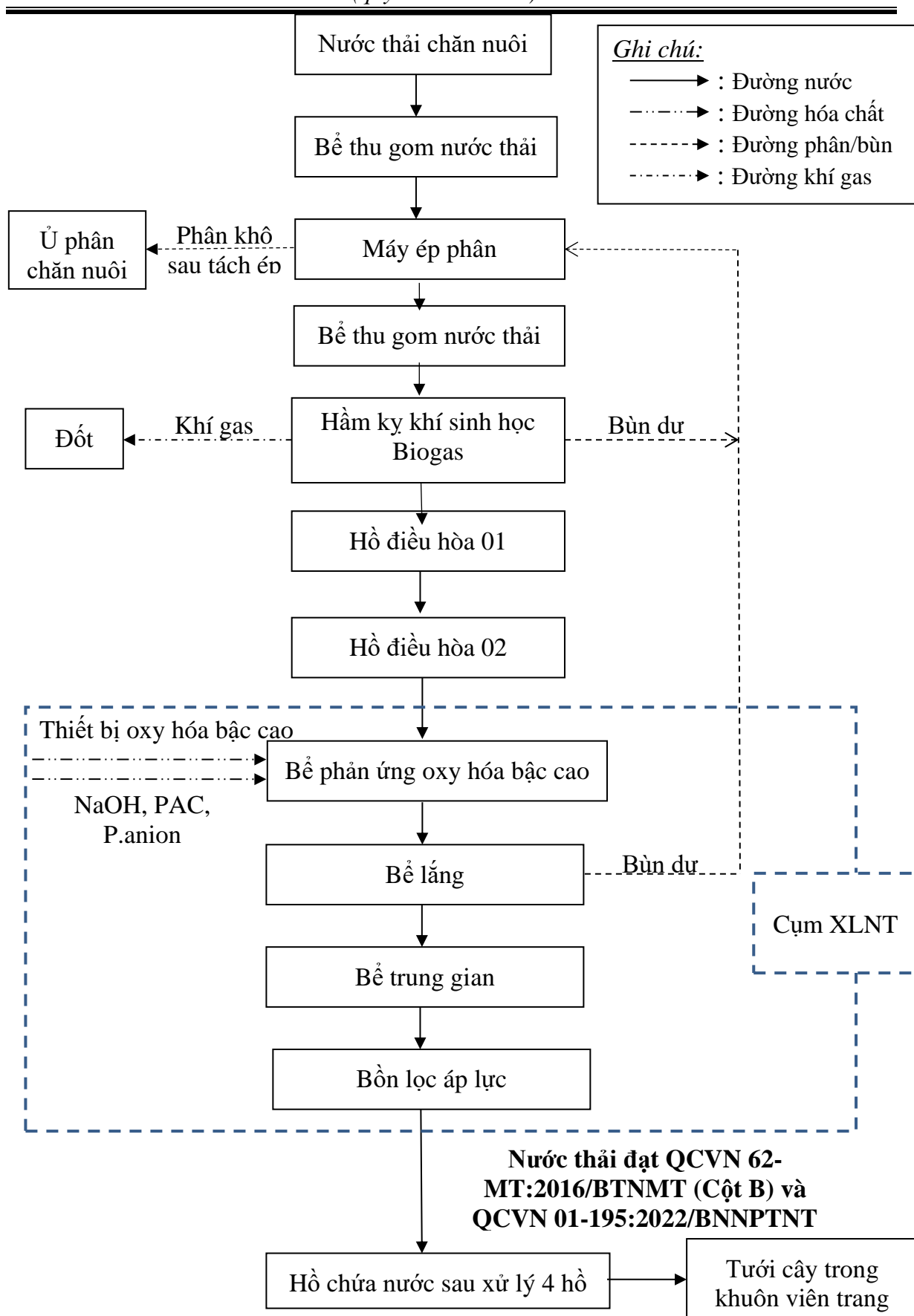
Hình 3.8: Sơ đồ công nghệ hệ thống xử lý nước thải tập trung của trang trại
